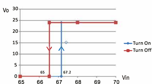
DDR-240D-24
