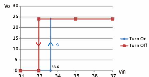
DDR-240C-24
