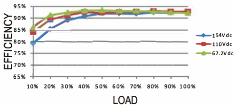
DDR-240D-24
